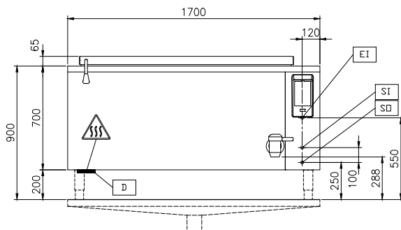
Front aanzicht
